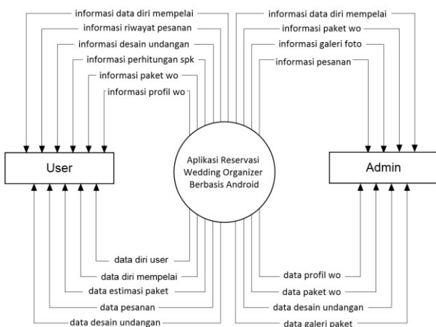
Gambar. 1.DAD Level 0
