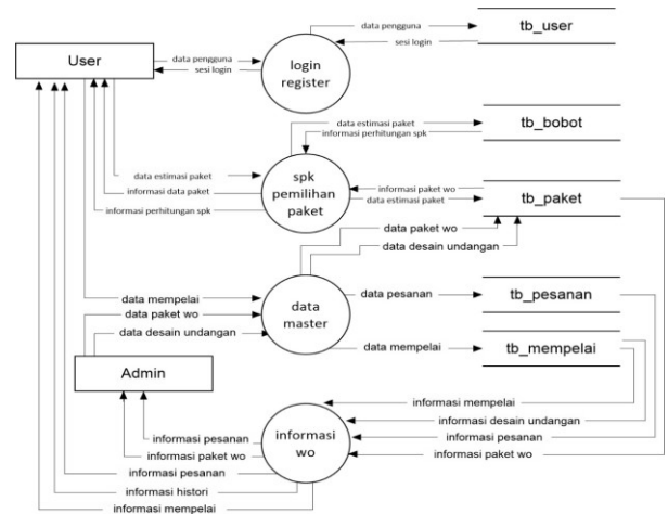
Gambar. 2.DAD Level 1
